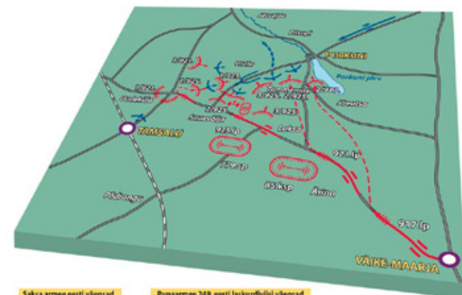
Lahingu skeem.
